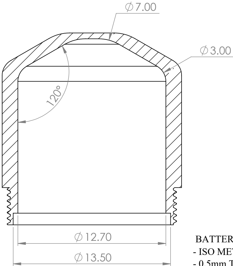
SECTION A-A
